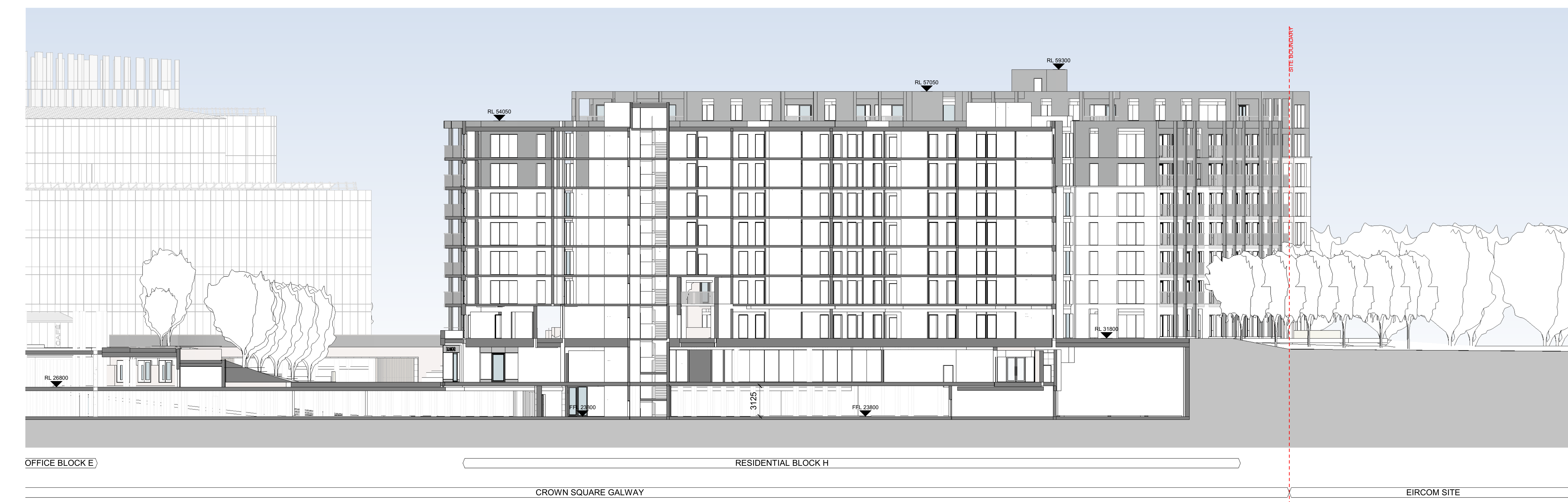
3 Site Section 11_1.200 1:200
